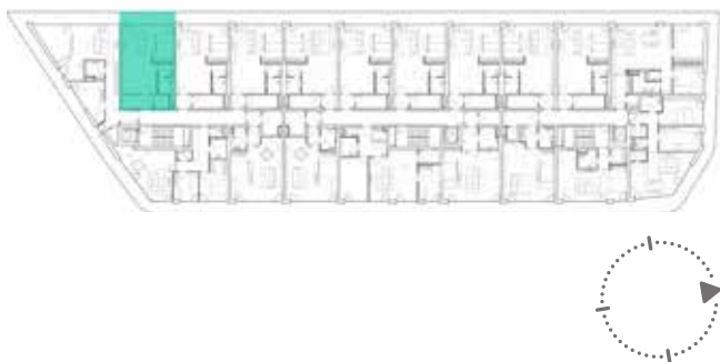
Plán podlaží
